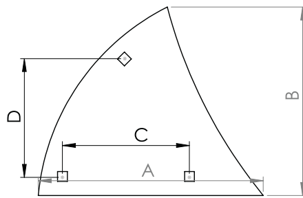
İKİLER LEMKEN AŞINMA PARÇASI / IK-YD-30-32223
